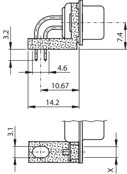
Kunststoffwinkel / Plastic bracket
