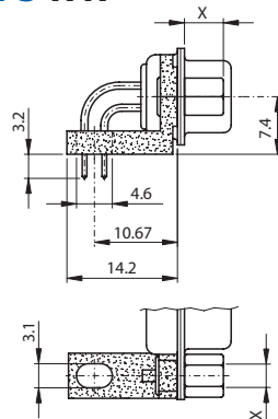
Kunststoffwinkel / Plastic bracket
