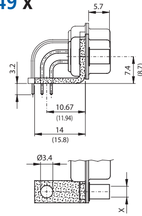
Metallwinkel / Metal bracket
